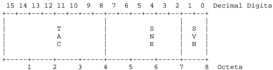
Figure 2: IMEISV Format
