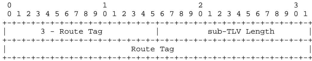
Route-Tag Sub-TLV
