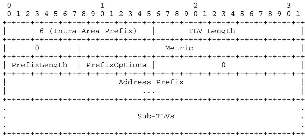
Intra-Area-Prefix TLV
