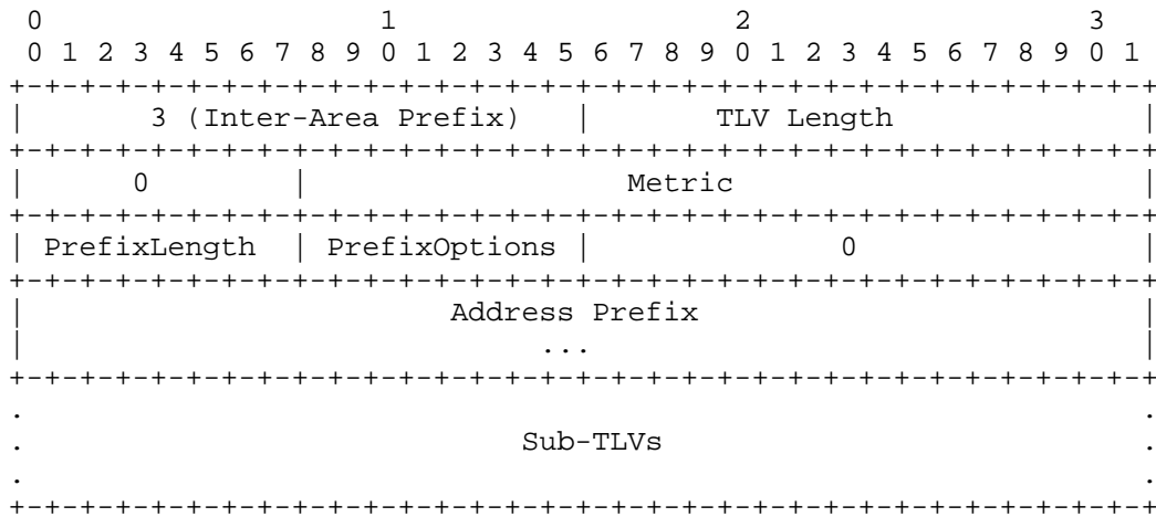
Inter-Area-Prefix TLV
