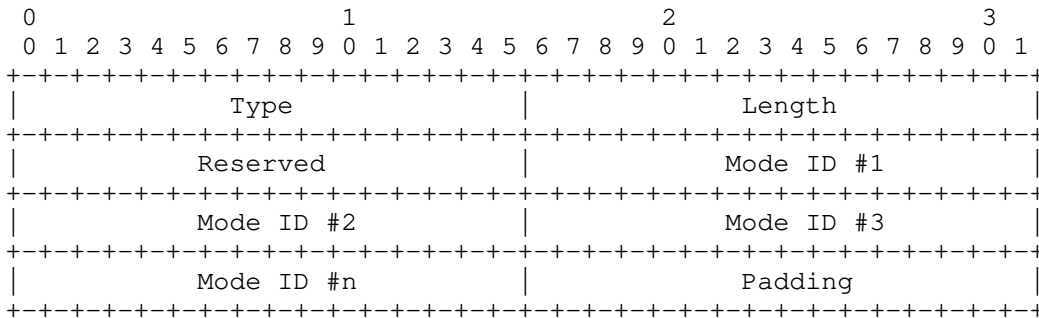
Figure 8: Format of the NAT_TRAVERSAL_MODE Parameter
