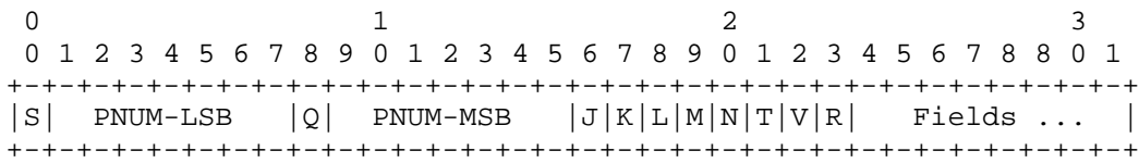
Figure A.4.2 -- Parameter Log Format
